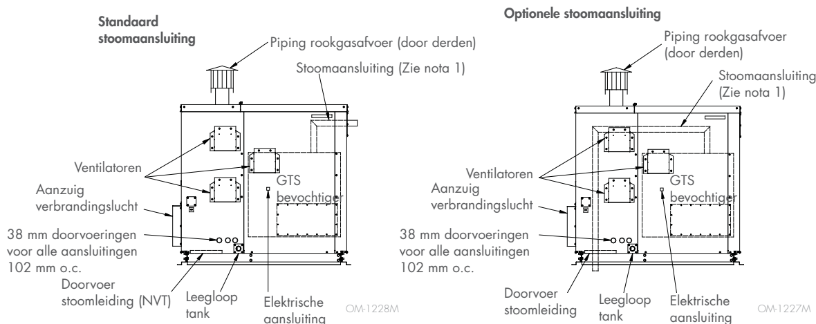
FIGURE 8-1: GTS BUITENOPSTELLING MET STANDAARD EN OPTIONEEL STOOMAANSLUITING, ZIJAAZICHT
