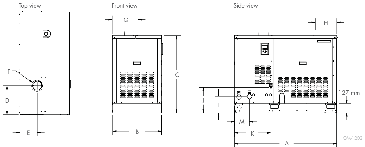
FIGUUR 6-1: AFMETINGEN
